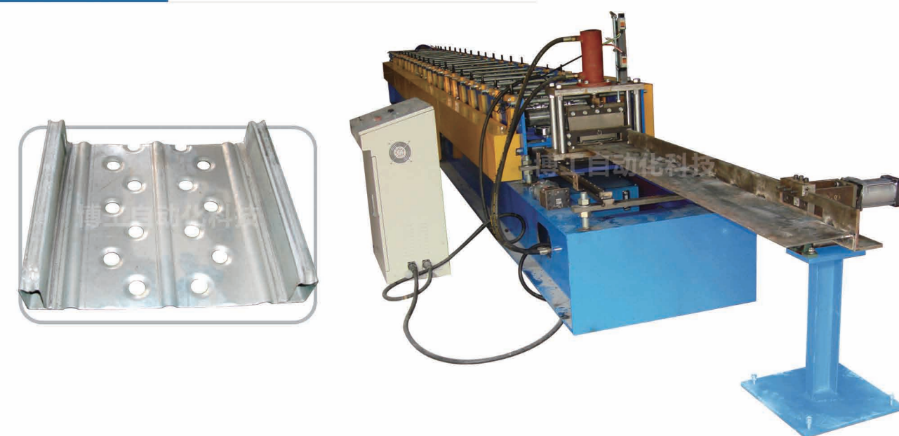
防滑板辊压成型机 Antiskid Plate Roll Forming Machine
