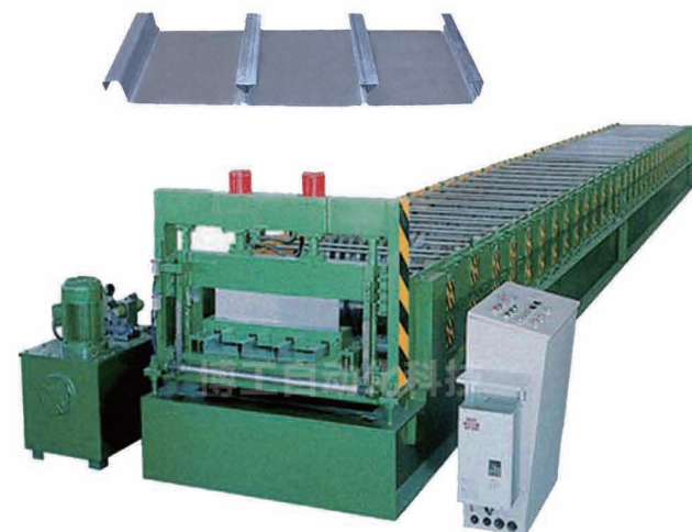
结构楼承板辊压成型机 Metal Deck Roll Forming Machine
